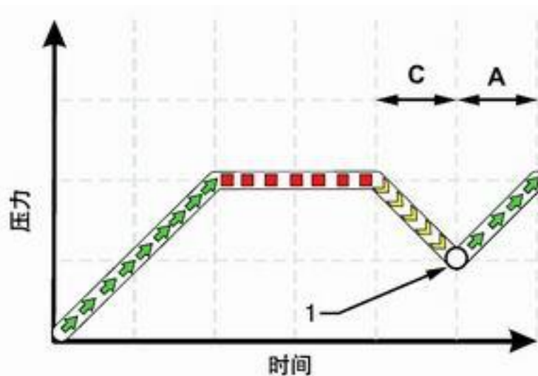
图 2-7 ABS 建压阶段曲线
