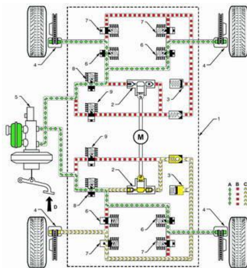
图 1-5 液压调节器总成内部液压回路示意图
