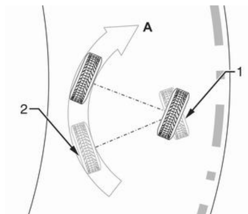
图 3-5 克服转向过度操作示意图
