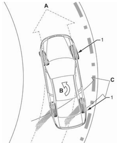
图 3-4 转向过度示意图
