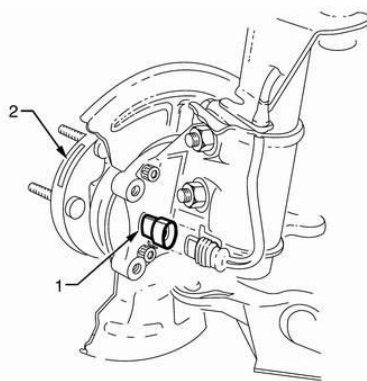
图 1-6 前轮速度传感器
