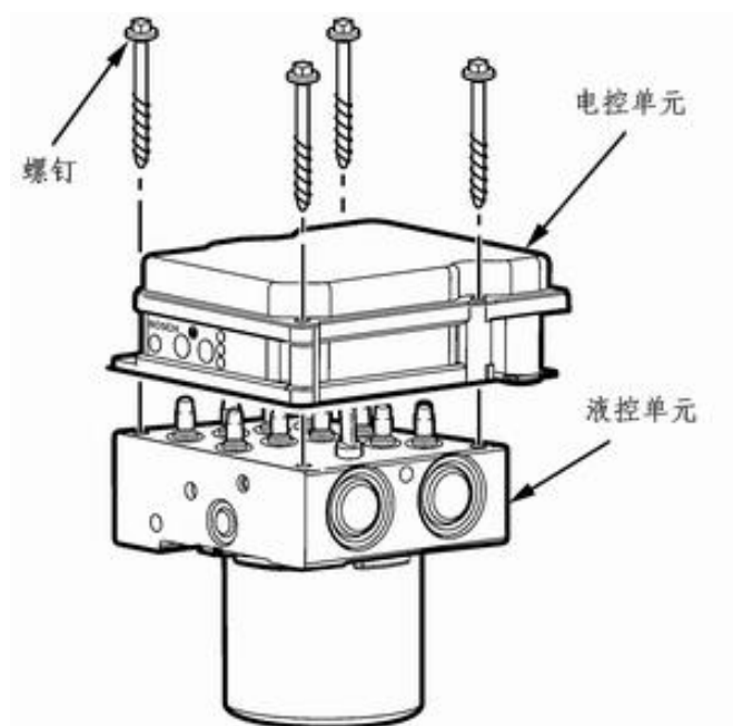
图 4-1 电子控制单元和液压总成
