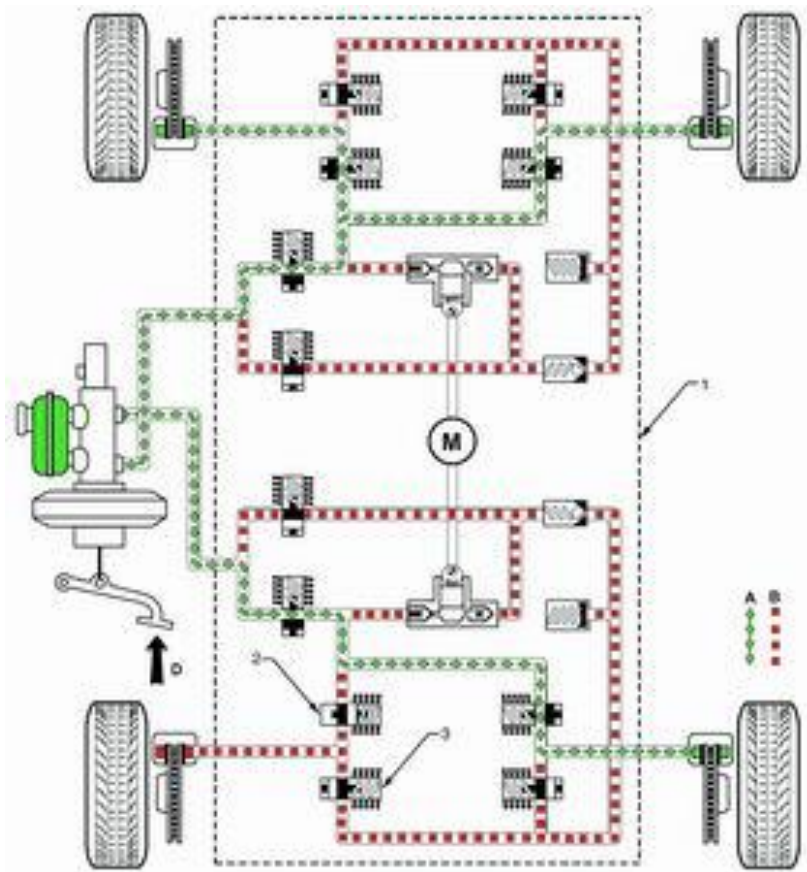
图 2-2 ABS 保压阶段控制油路
