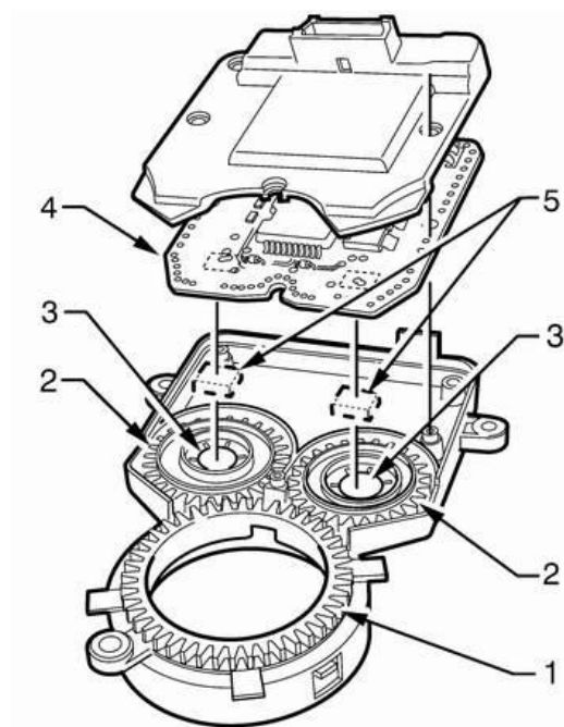
图 1-10 方向盘转角传感器
