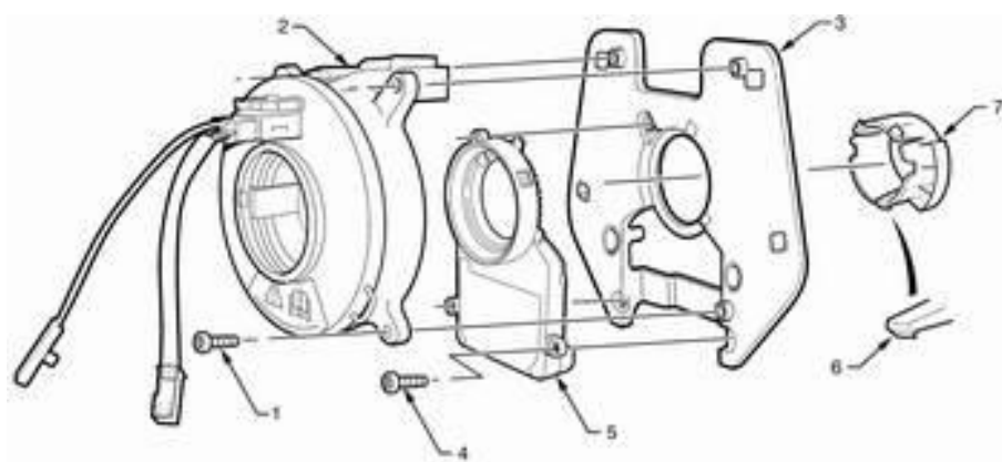
图 1-9 方向盘转角传感器的位置
