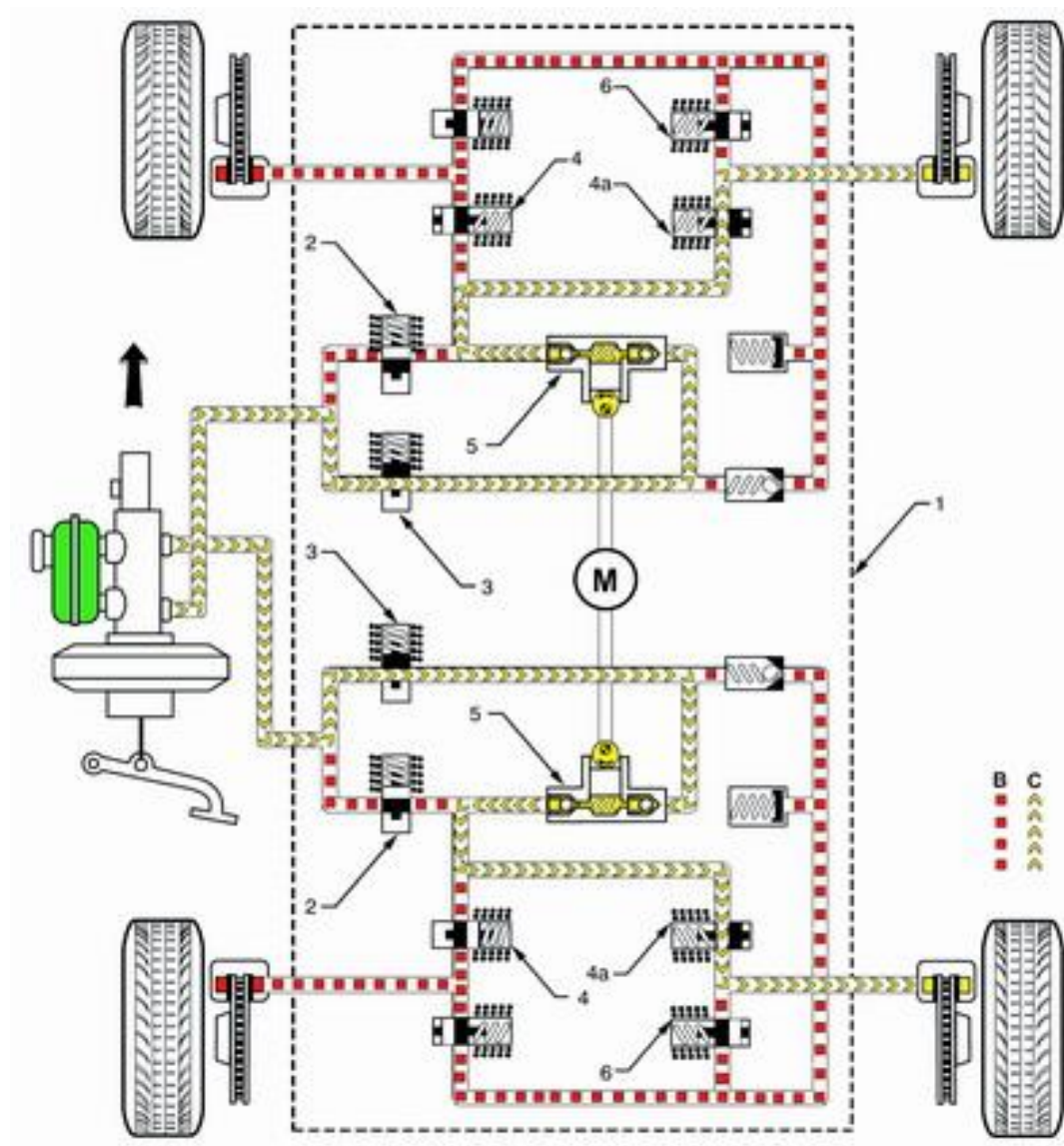
图 3-6 克服转向过度控制油路图
