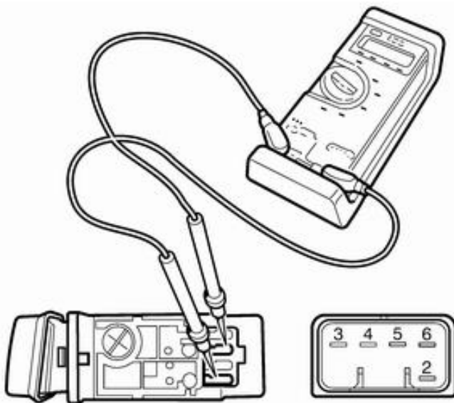
图 4-2 ESP 开关端子视图及检查方法
