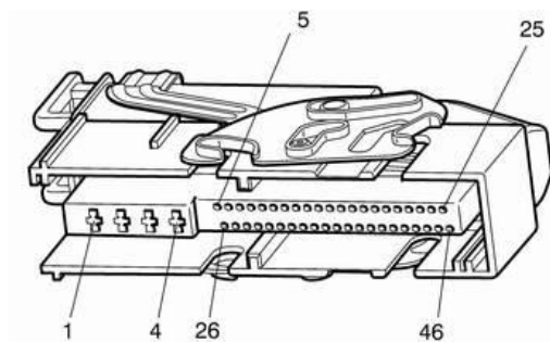
图 1-4 电子控制单元 (ECU) 插头端子视图
