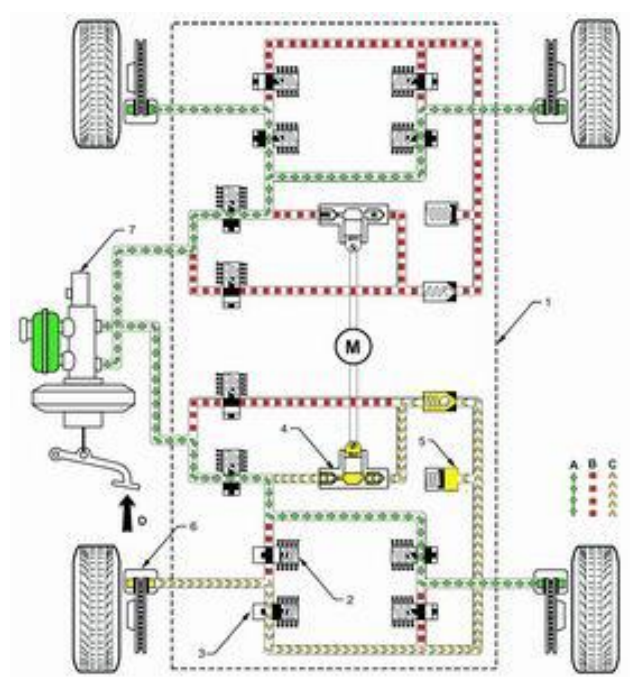
图 2-4 ABS 减压阶段控制回路
