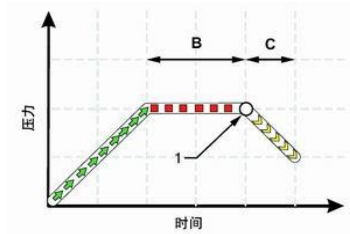
图 2-5 ABS 减压阶段曲线图
