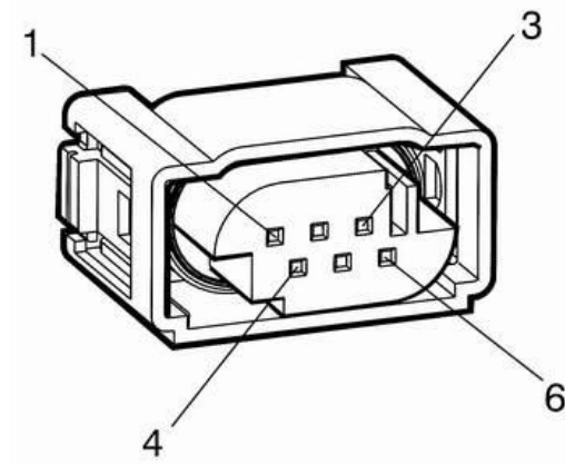
图 1-13 横向偏摆率传感器插头端子视图
