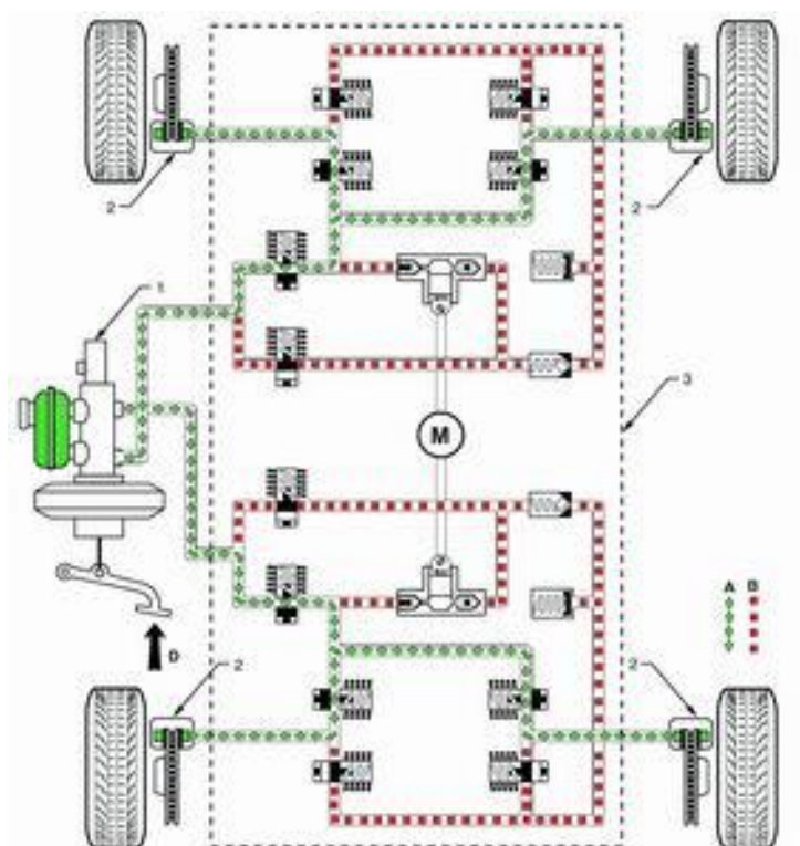
图 2-1 常规制动控制油路
