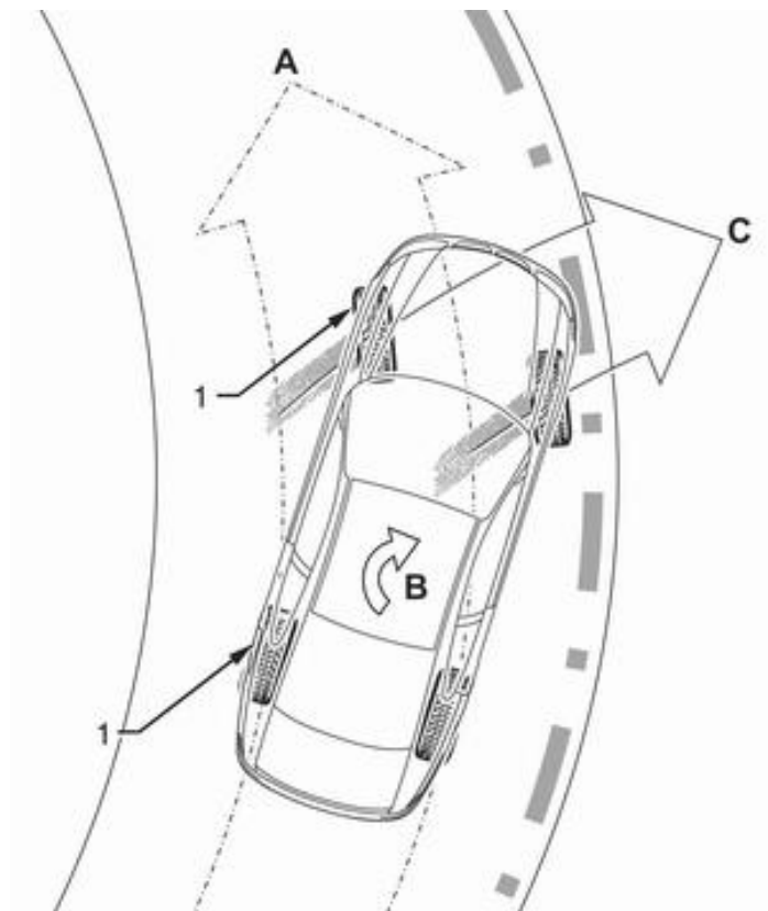
图 3-1 转向不足示意图
