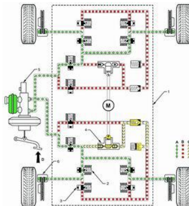
图 2-6 ABS 建压阶段控制回路
