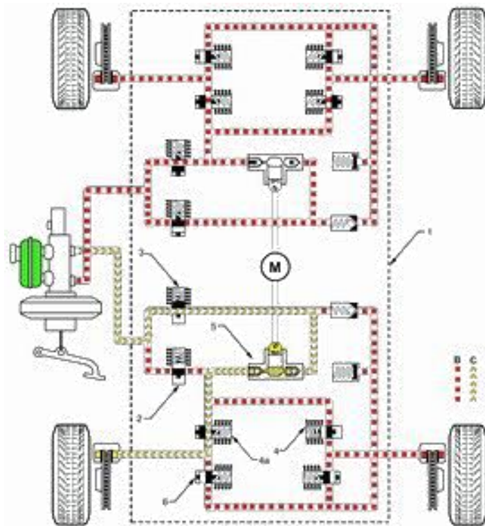
图 2-8 TCS 制动干预（以左后轮为例）
