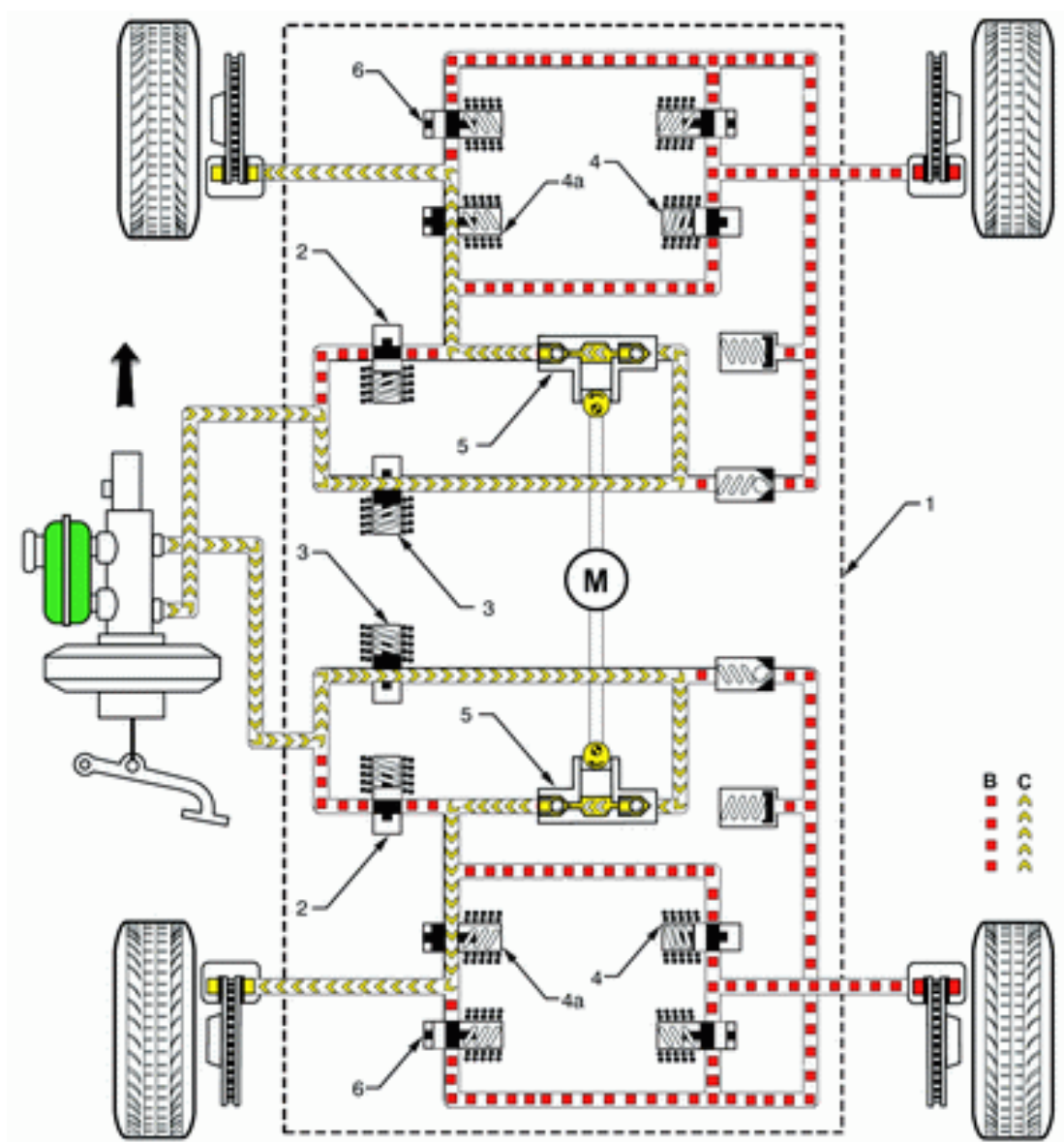
图 3-3 克服转向不足控制油路图
