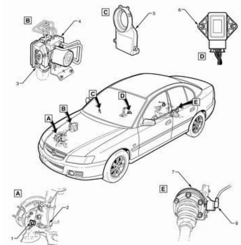
图 1-1 奔驰轿车电子制动系统的组成图
